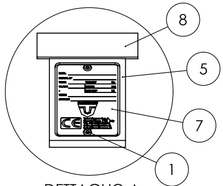
DETTAGLIO A SCALA 1 : 3
